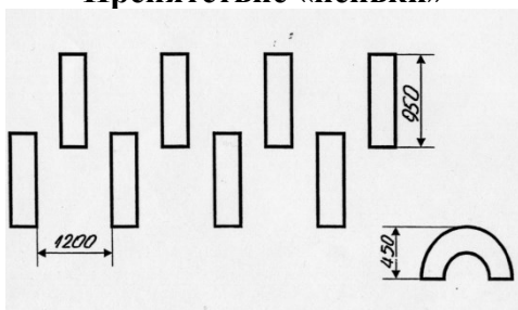
Препятствие «пеньки»
