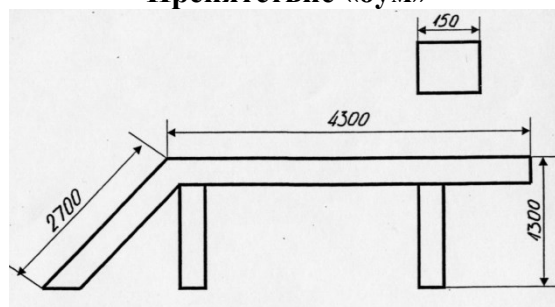
Препятствие «бум»
