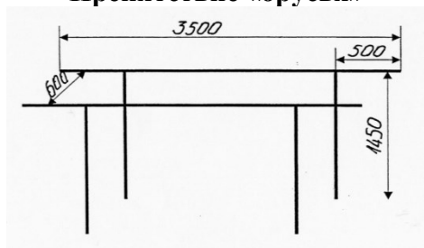
Препятствие «брусья»
