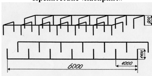
Препятствие «лабиринт»
