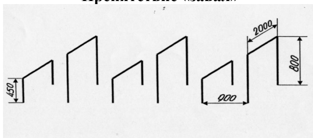
Препятствие «завал»
